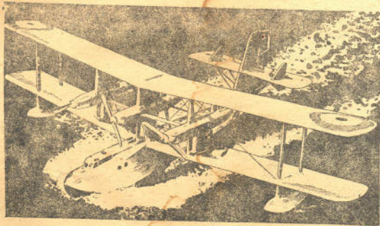
მსოფლიოში უდიდესი სამხედრო გიდროპლანი, რომელიც ეკუთვნის ინგლისს, მთლიანად ლითონიდანაა დაზადებული. მასზე დადგმულია ექვსი 880 ძალისანი მო- ტორი, შეუძლია 33 ტონა მასალის წაღება.
