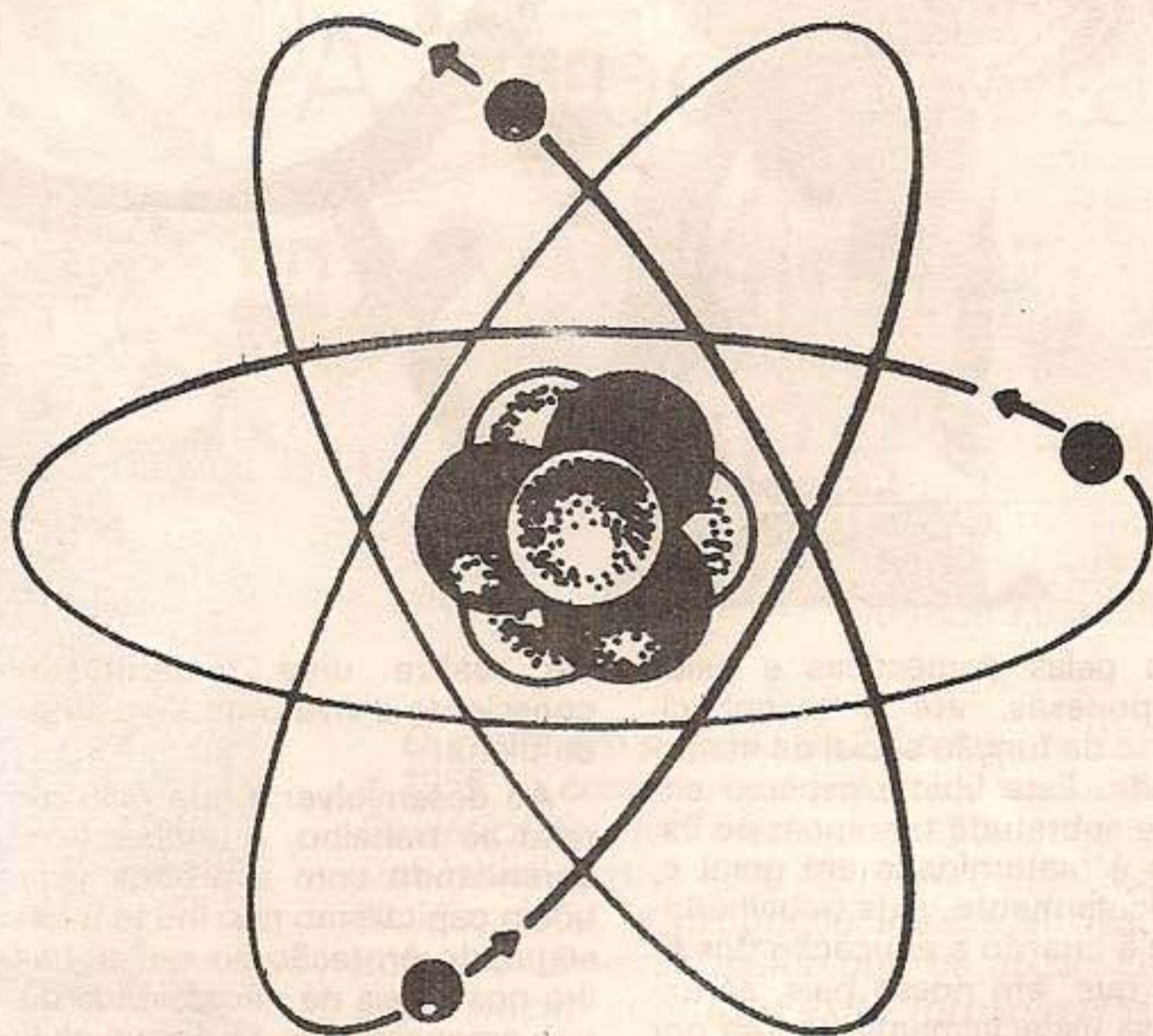
Um modelo simples da estrutura de um átomo.
